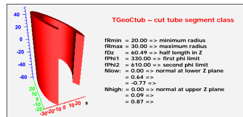
Figure 19-11 TGeoCtub Class
