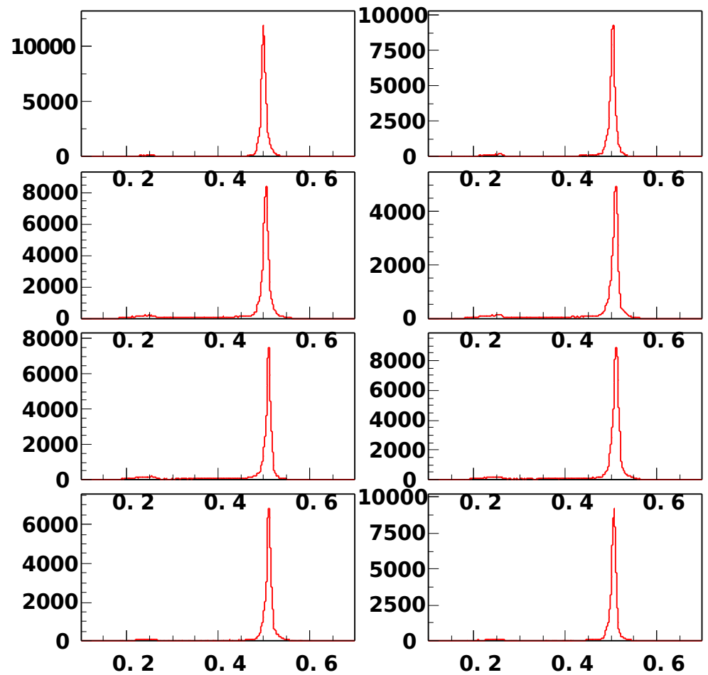
Positrons
